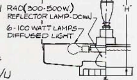
LAMPING DIAGRAM CPI-343-30
