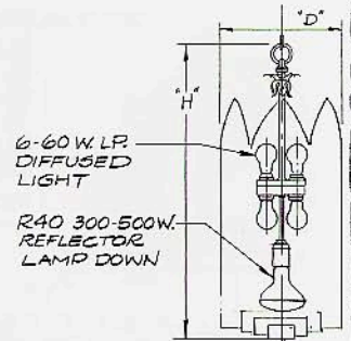
LAMPING DIAGRAM LPI-353-13
