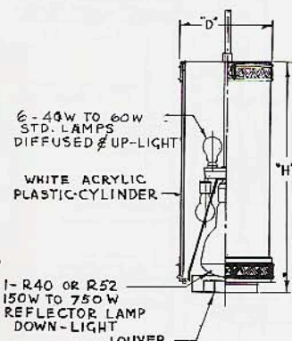
LAMP DIAGRAM-LPI-346-12
